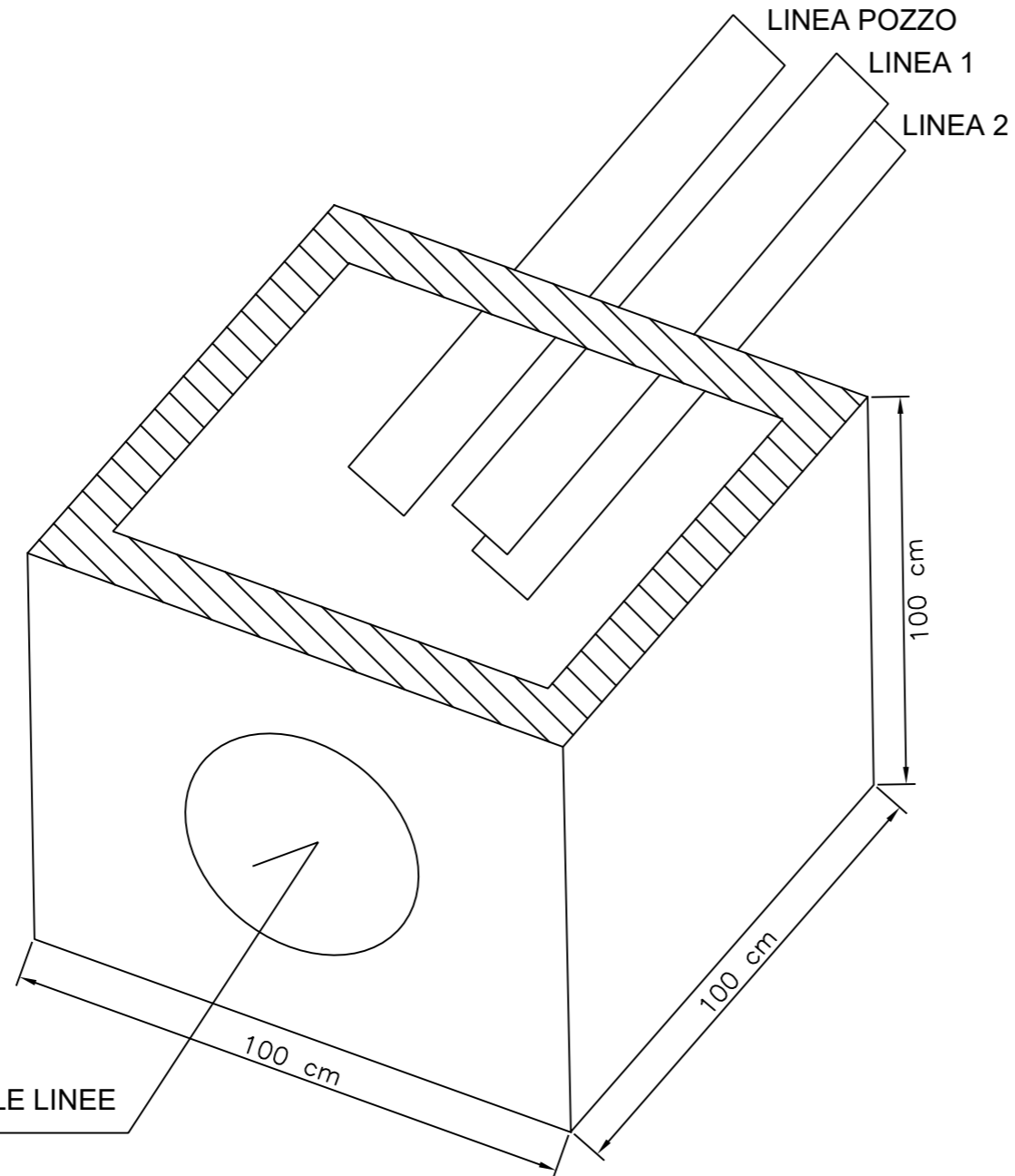
DISPOSIZIONE TIPO TUBI COLLETTAMENTO LINEA 1
